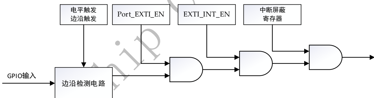
图 4-1 EXTI 系统框图
