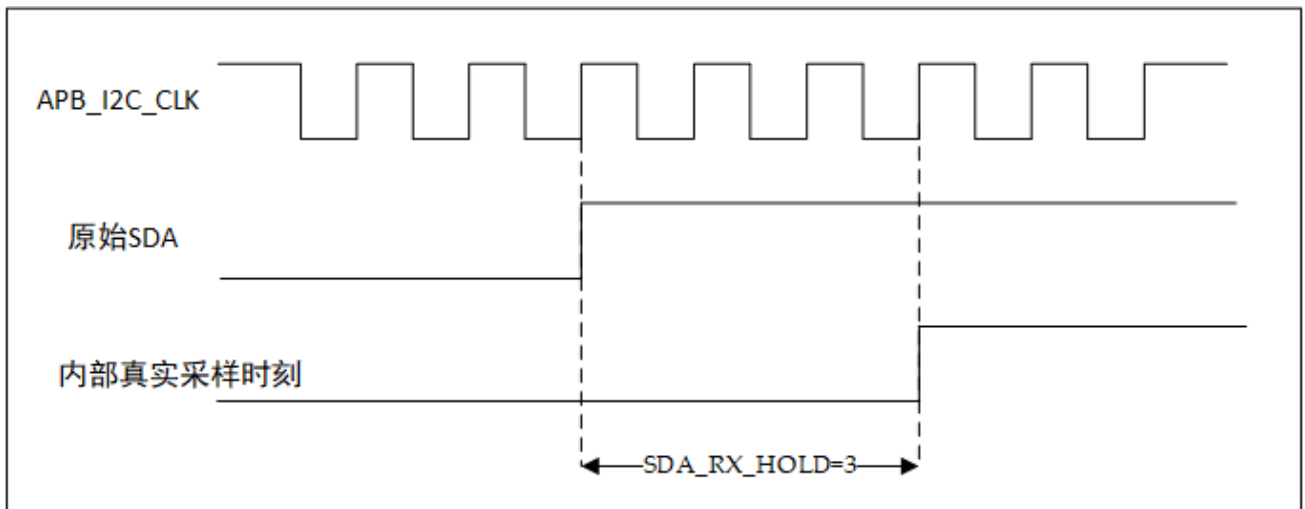
图 8-3 SDA_RX_HOLD 使用示意图
