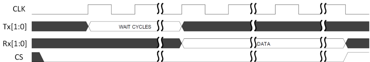
图 6-9 读数据，没有指令，没有地址，仅数据传输
