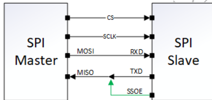
图 6-1 SPI Master 接线示意图
