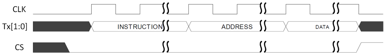
图 6-4 指令、地址和数据使用多线模式
