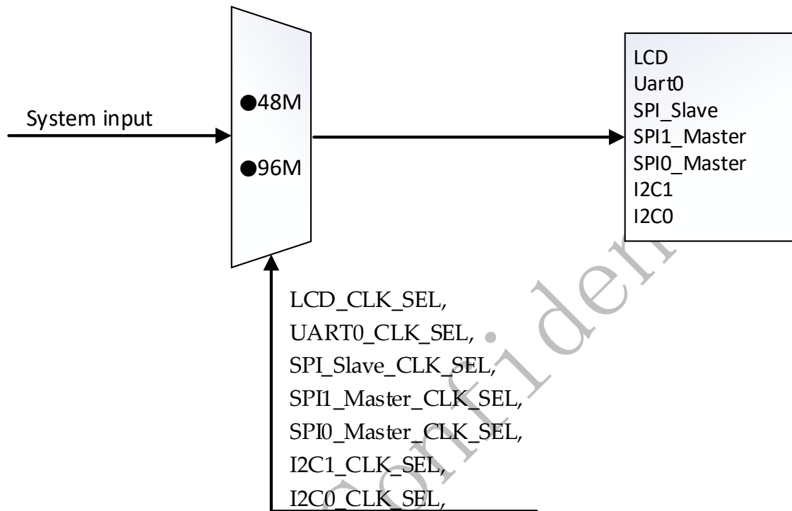
图 2-2 外设时钟配置
