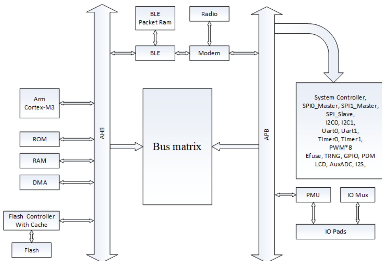
图 1-1 系统框图
