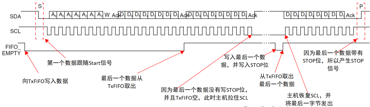
图 8-9 主机发送并产生 STOP
