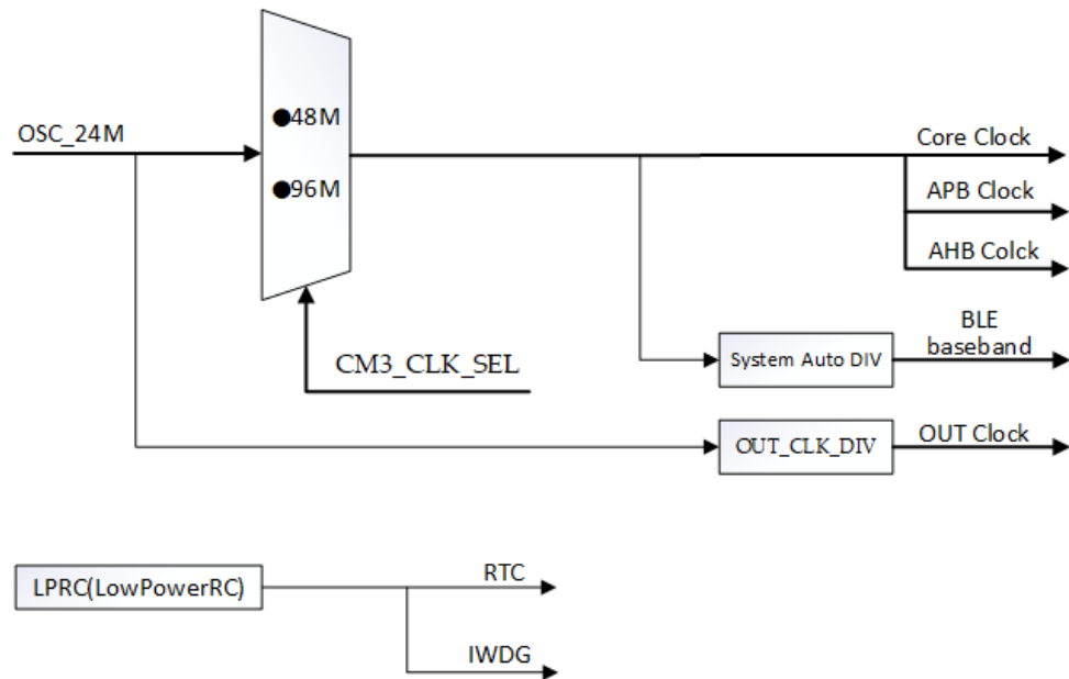
图 2-1 系统时钟树
