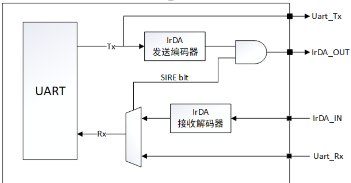
5-1 IrDA 框图
