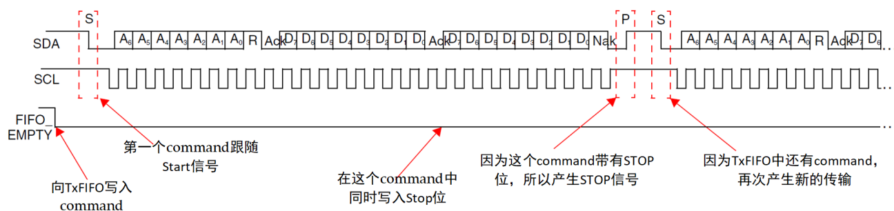
图 8-14 主机接收，产生 STOP，TxFIFO 非空
