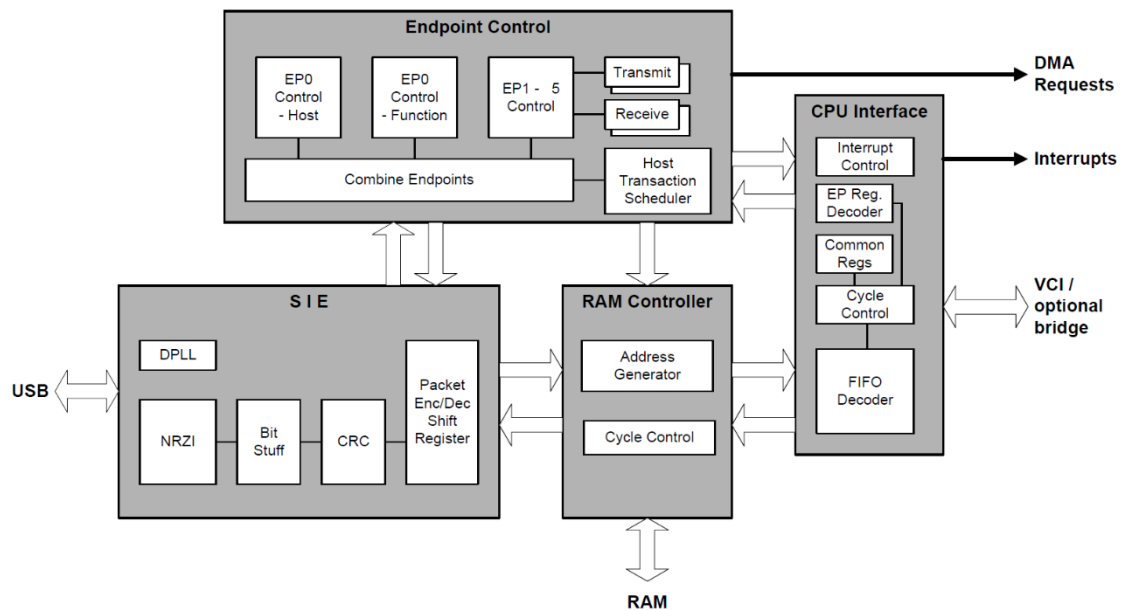
图 18-1 USB 系统框图
