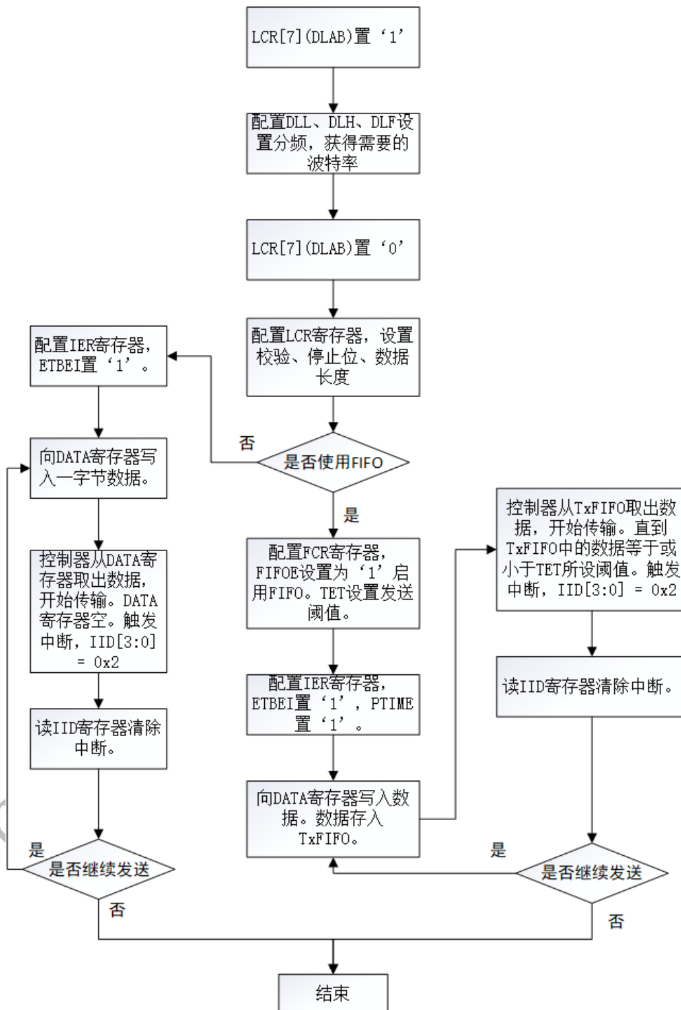
图 5-3 发送数据流程
