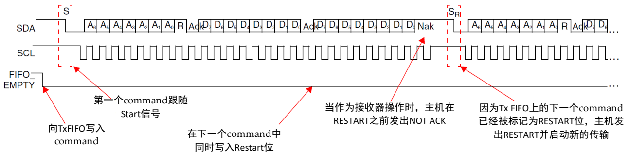
图 8-12 主机接收并产生 Restart 时序
