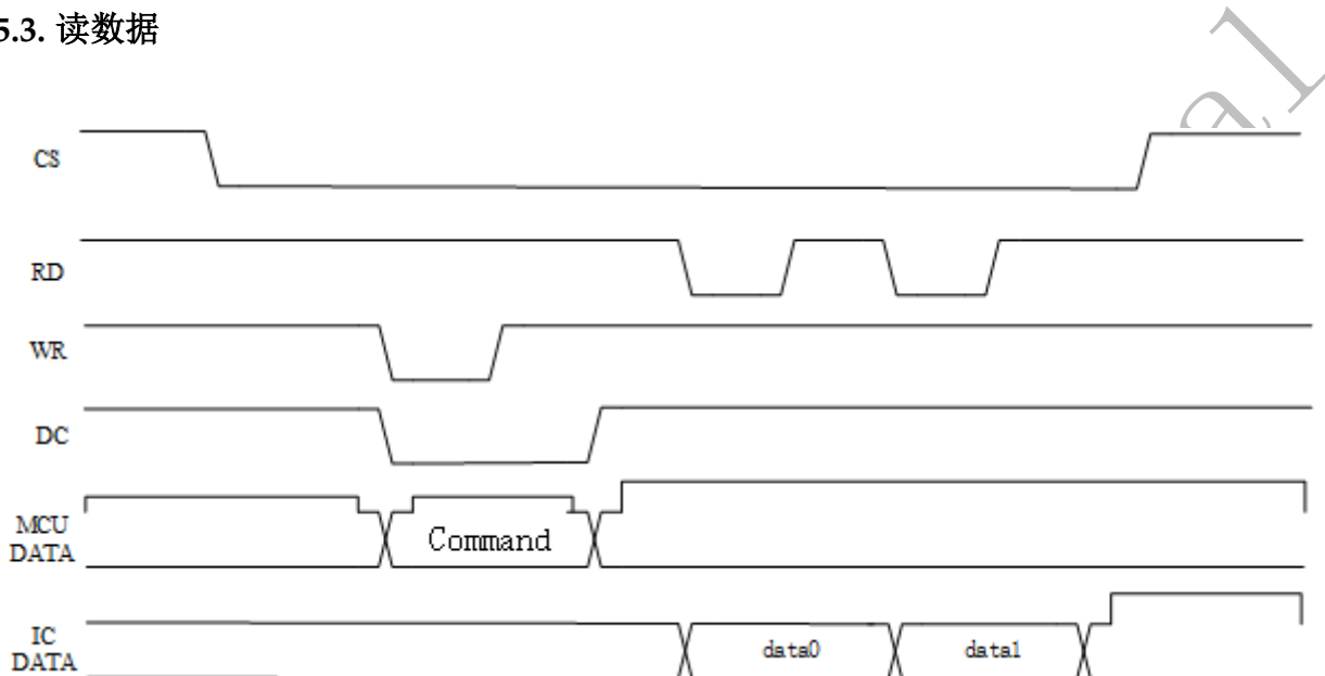
图 15-4 8080 读数据时序
