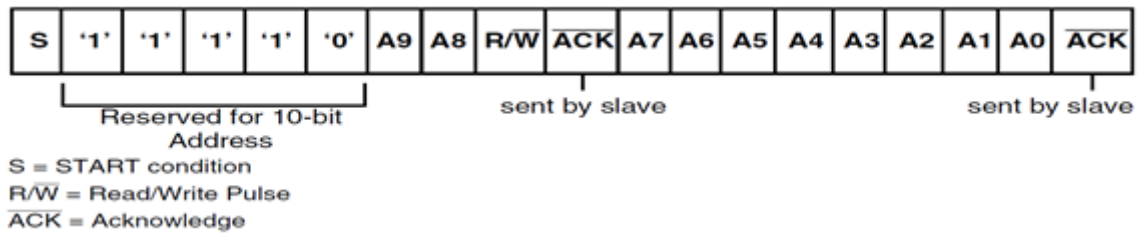
图 8-6 10bit 地址示意图
