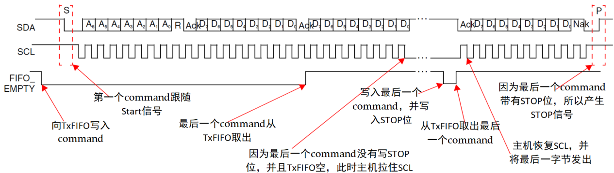
图 8-10 主机接收并产生 STOP 时序
