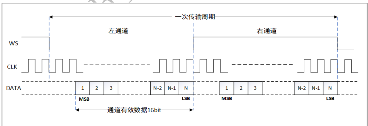
图 9-4 I2S 时序图（左对齐，WS 反相，DLY_EN = 1）
